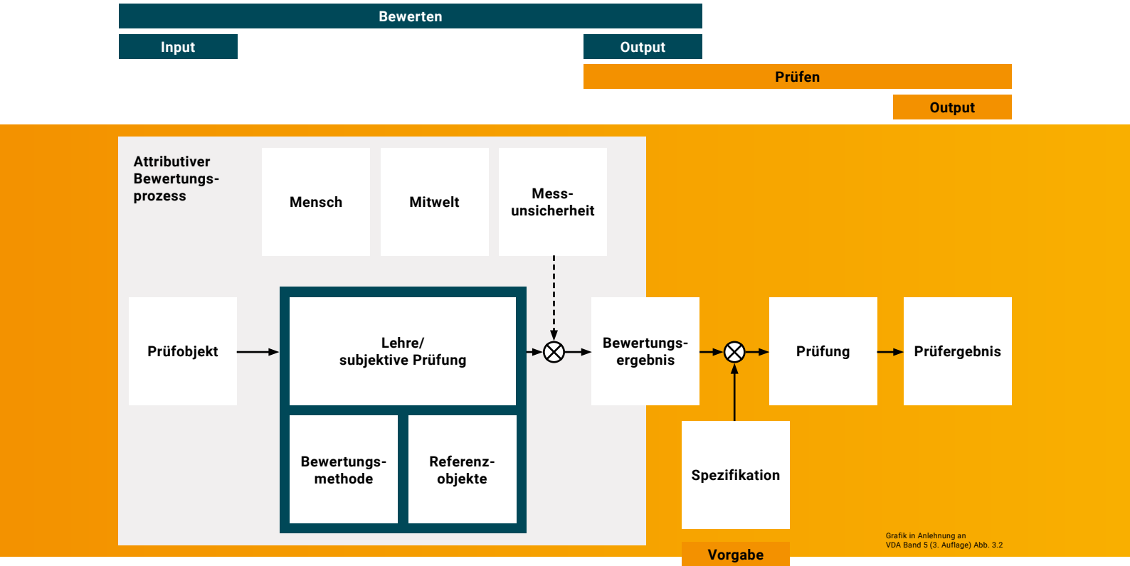
Abbildung 2: Attributiver Prüfprozess
