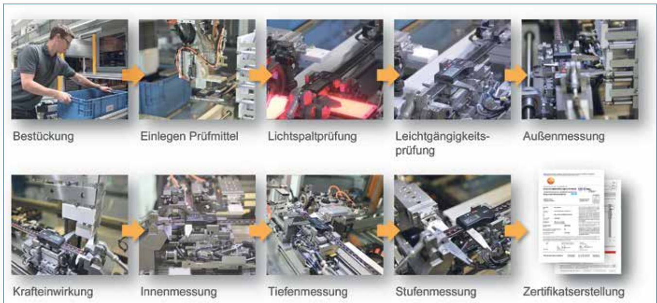
Bild 1. Von der Bestückung bis zum Zertifikat: Ablauf einer voll automatisierten Kalibrierung eines Messschiebers
